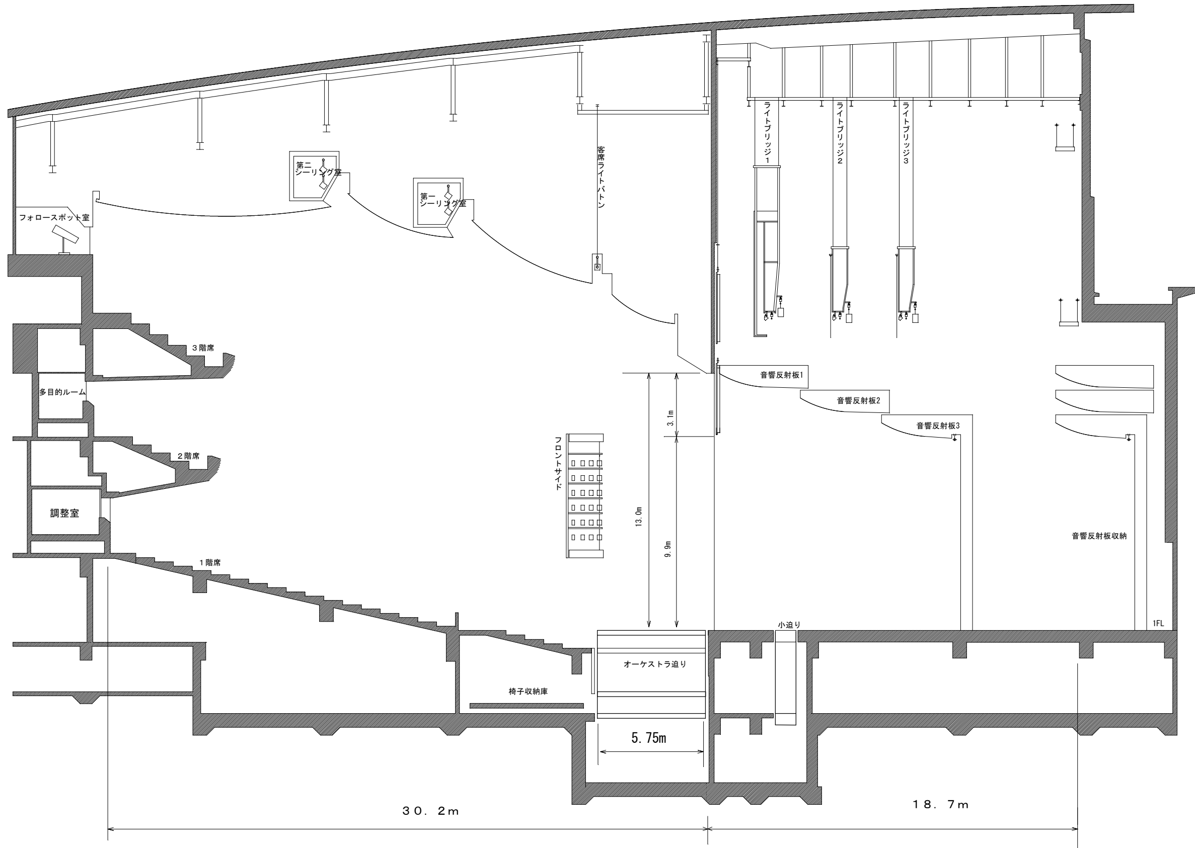
鳥取県立倉吉未来中心 大ホール断面図 (1:200 A3)
