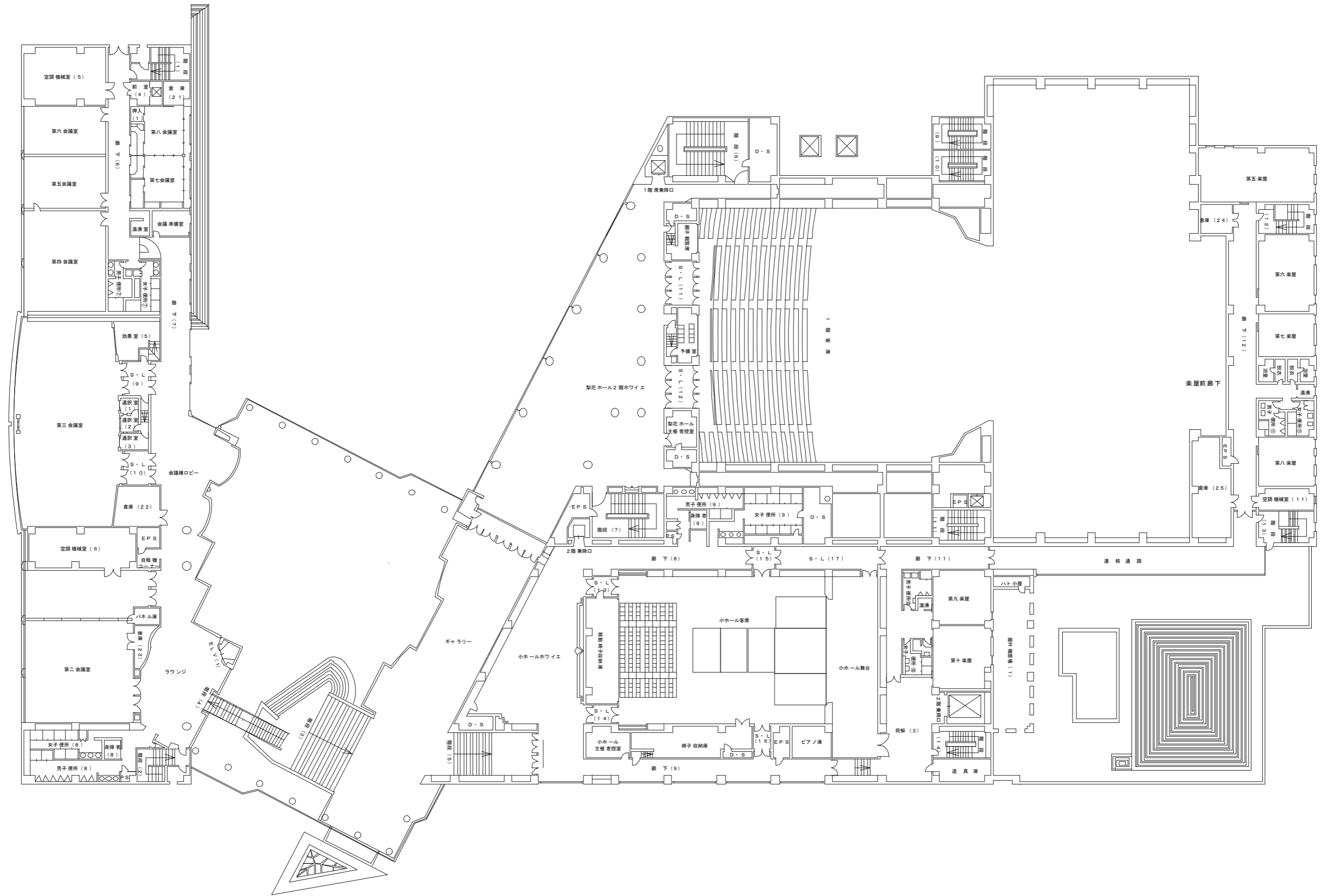
2階平面図
